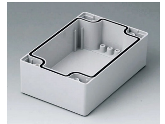
C2081202 Gehäuseschale 80, mit Dichtung PC (UL 94 HB) lichtgrau RAL 7035 120x80x40mm
