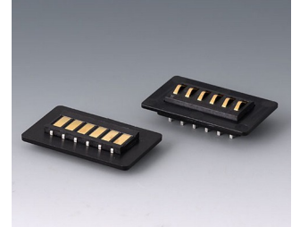
A9193044 Kit fiches modulaires à 6 contacts ABS (UL 94 HB) noir RAL 9005
