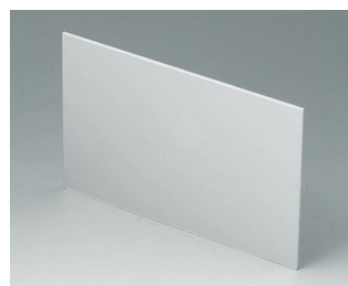
A9114221 Лицевая / задняя панель V, O 190 Алюминий матово-анодированный 124,2x79,6x1,5mm
