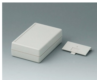
A9406352 SHELL-TYPE CASE G 110, исп. II ABC (UL 94 HB) белый RAL 9002 72x114x33,5mm
