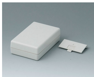
A9406332 SHELL-TYPE CASE G 110, исп. II АБС (UL 94 HB) белый RAL 9002 72x114x33mm
