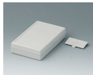
A9408355 SHELL-TYPE CASE G 155, исп. IV ABC (UL 94 HB) белый RAL 9002 95x158x33,5mm
