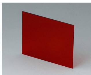
A9106223 Лицевая / задняя панель V 110 Алюминий прозр. красная 59,3x49x1mm
