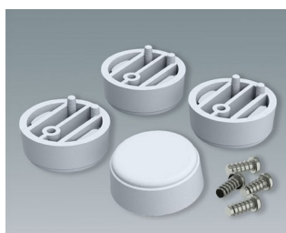
A9257405 Ножки для корпуса, исп. I АБС (UL 94 HB) светло-серый RAL 7035 ø30x12mm
